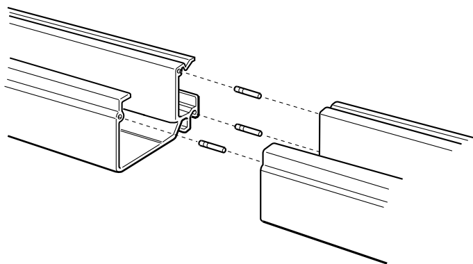
Bild 4. Skarvning av löpskena
