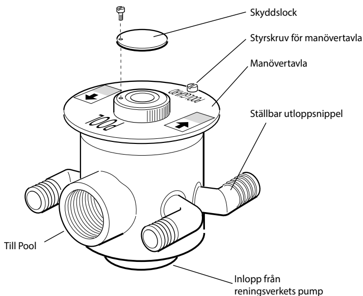
Bild 18. Shuntventil
