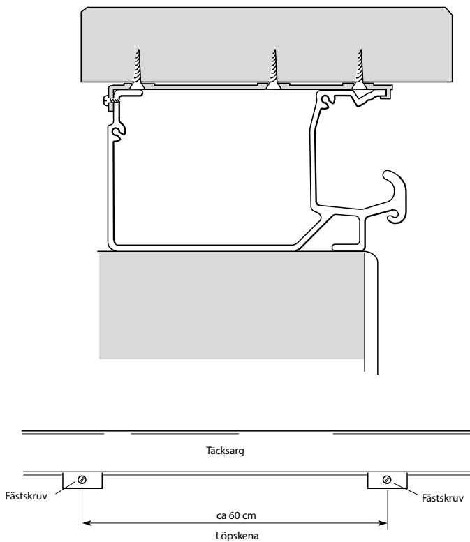
Bild 31. Montering av träsg
