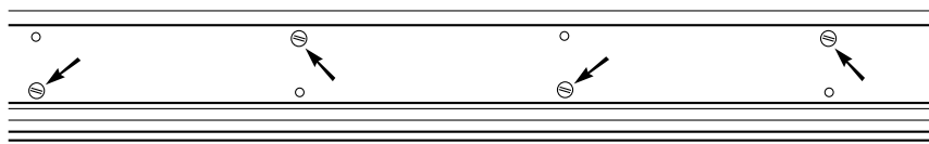
Bild 6. Löpskenans fästsruvar, typ U-skena
