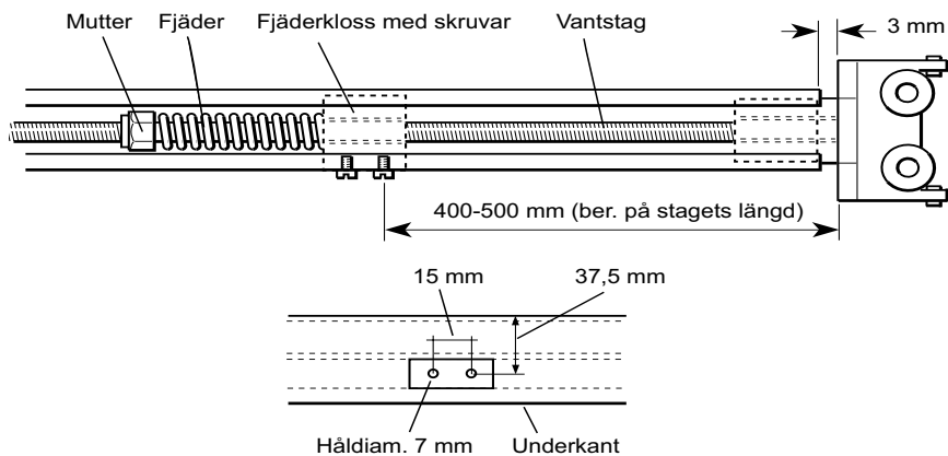
Bild 9b. Renkapning av fronskenan
